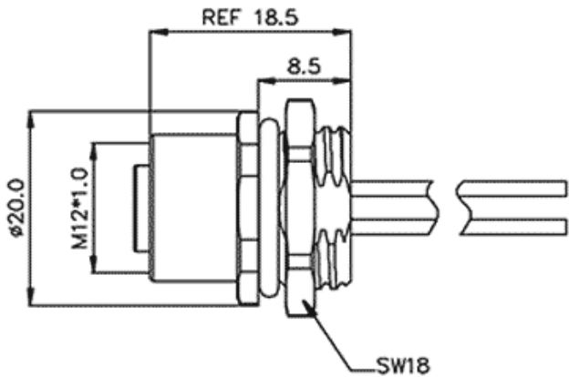
PG9 安装尺寸 Installation dimension
