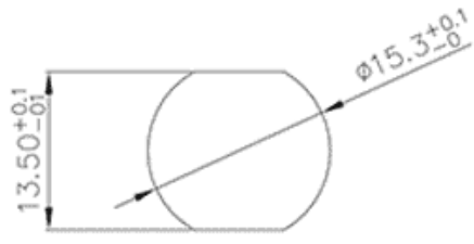
PG9 安装尺寸 Installation dimension
